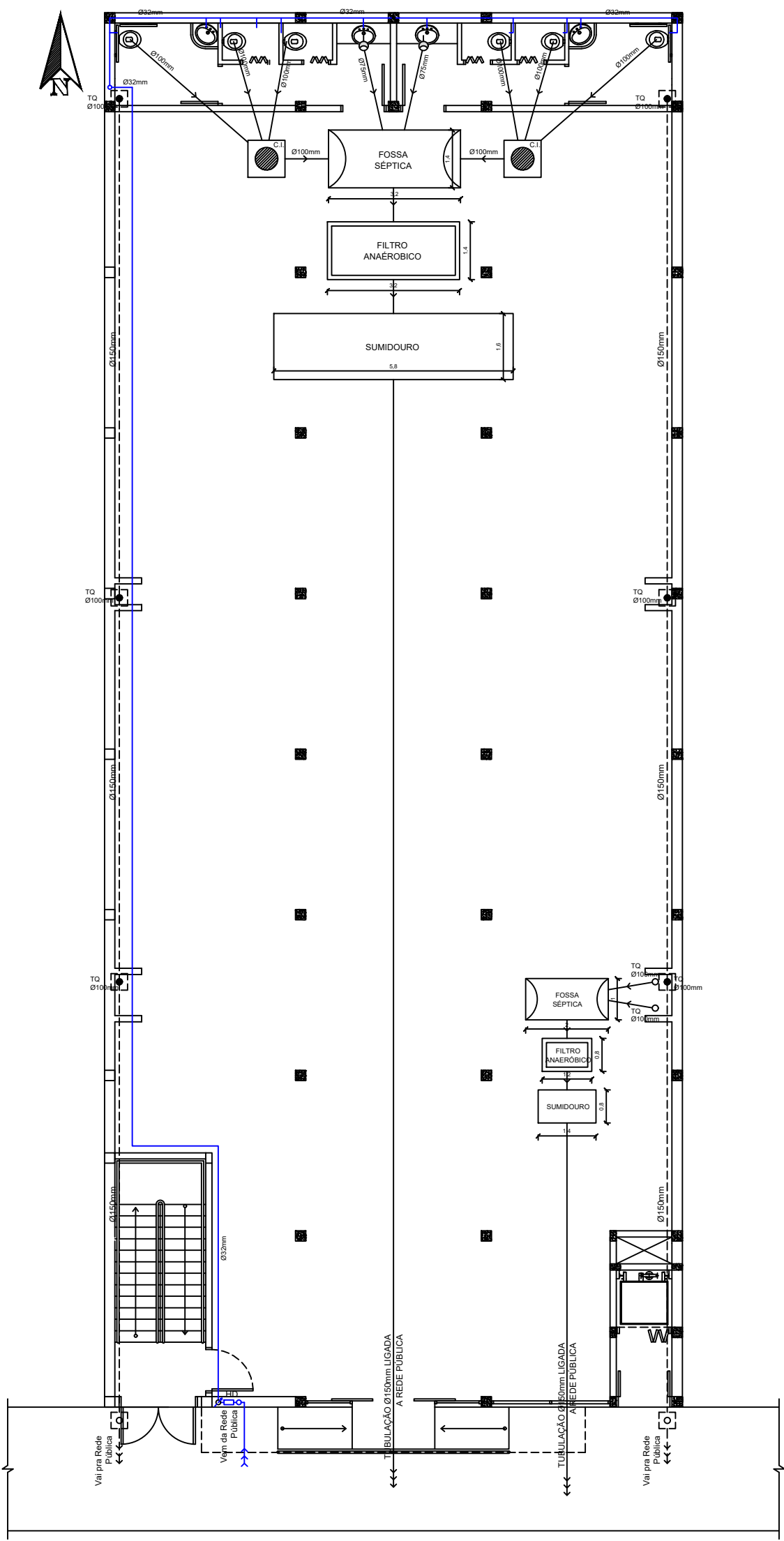
PLANTA DE INST. HIDROSSANTÁRIAS Esc: 1/75
