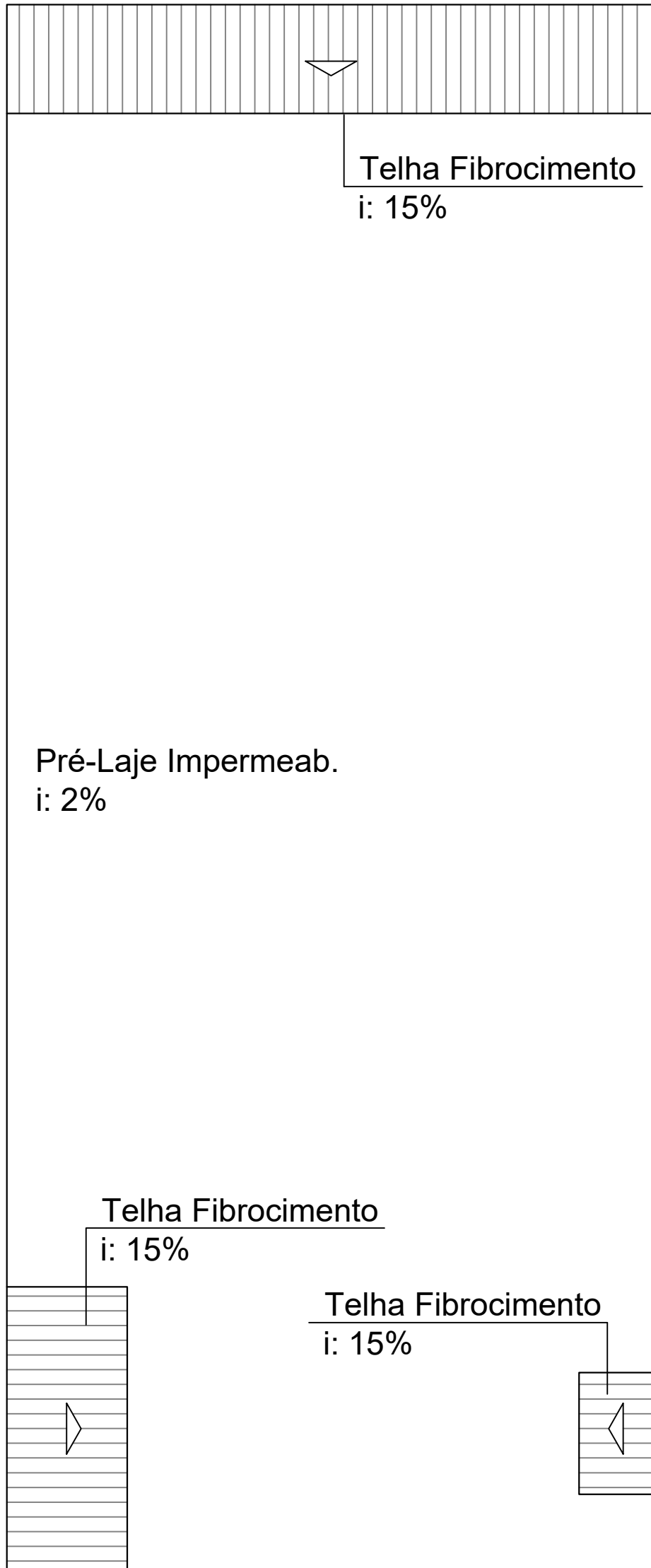
PLANTA DE COBERTURA Esc: 1/75
