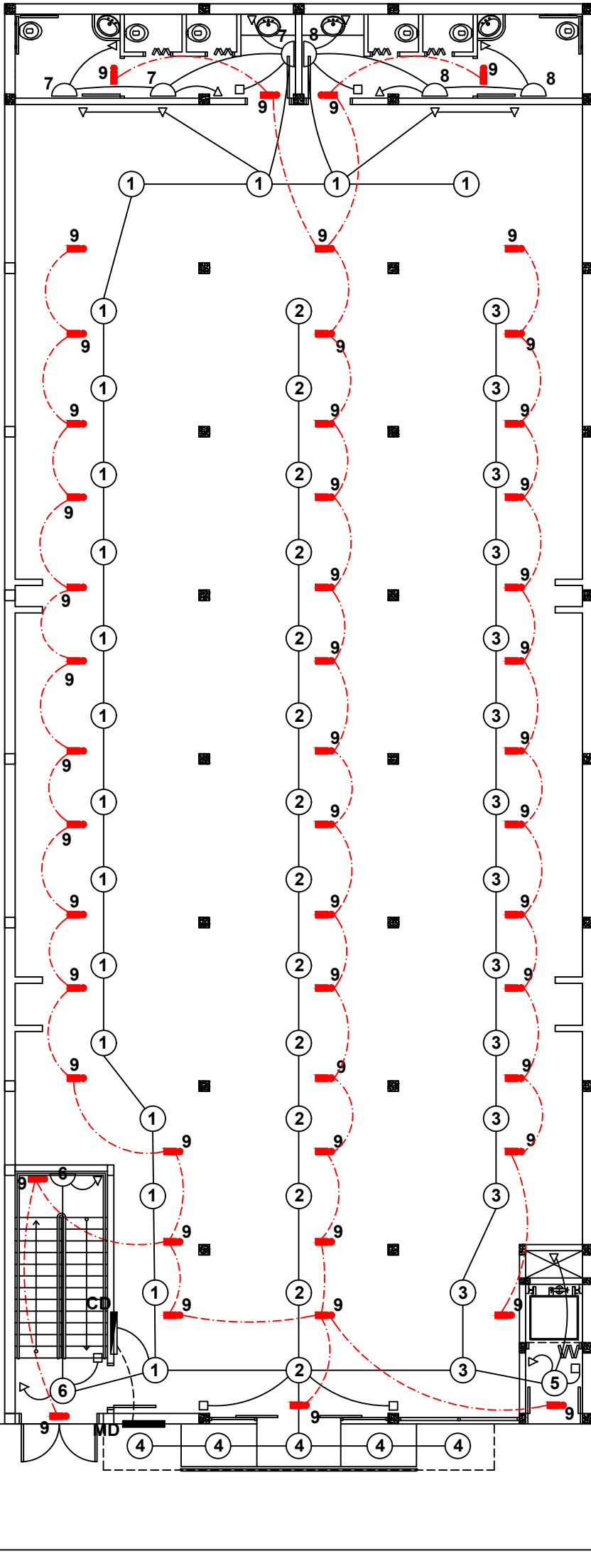
PLANTA DE INST. ELÉTRICAS Esc: 1/75
